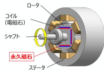
代表的な電気モータの構造
