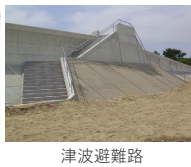
津波避難路
