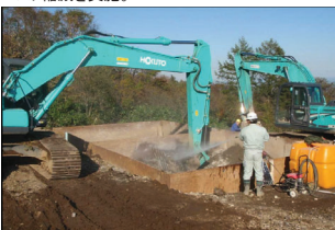
現場発生材を使用した砂防ソイルセメント工法による打設
