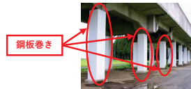
鋼板巻きによる耐震補強
