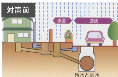
下水の排除方式 (合流式)
