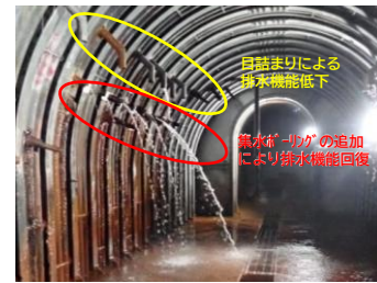
集水ボーリングの追加
