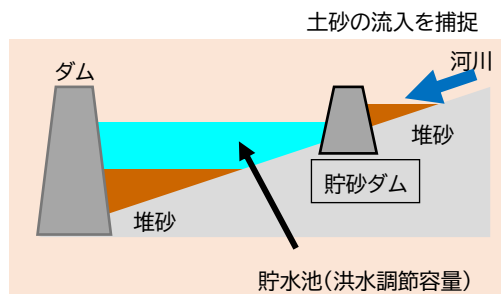
貯砂ダムによる効果イメージ図
