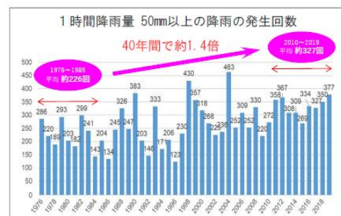
【短時間強雨の発生回数】
