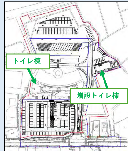
道の駅図面
