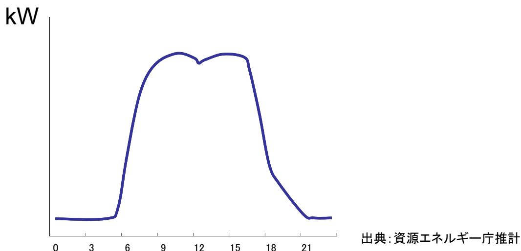
図1：公立小学校（事例）における電力需要カーブのイメージ（就学日）
