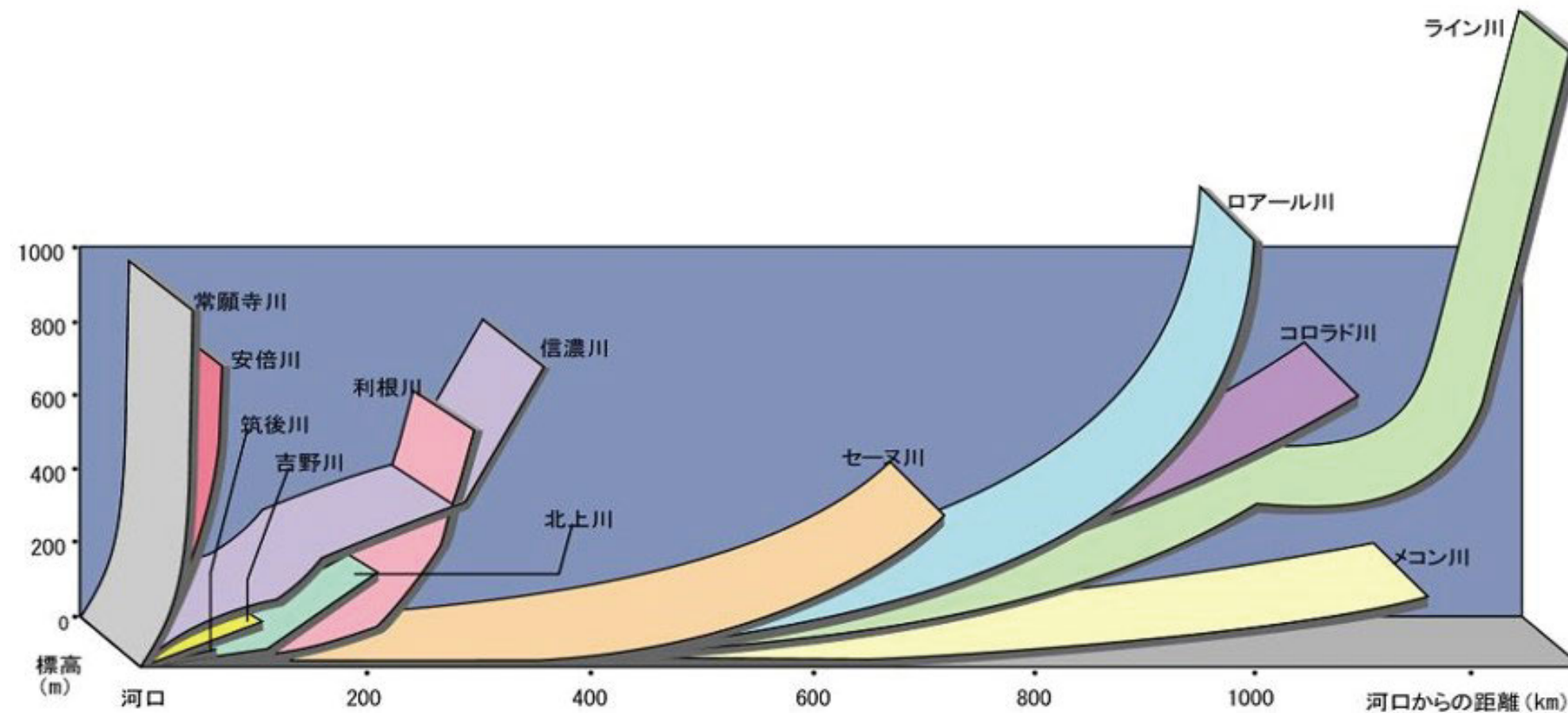
各国及び我が国の主要な川の勾配
