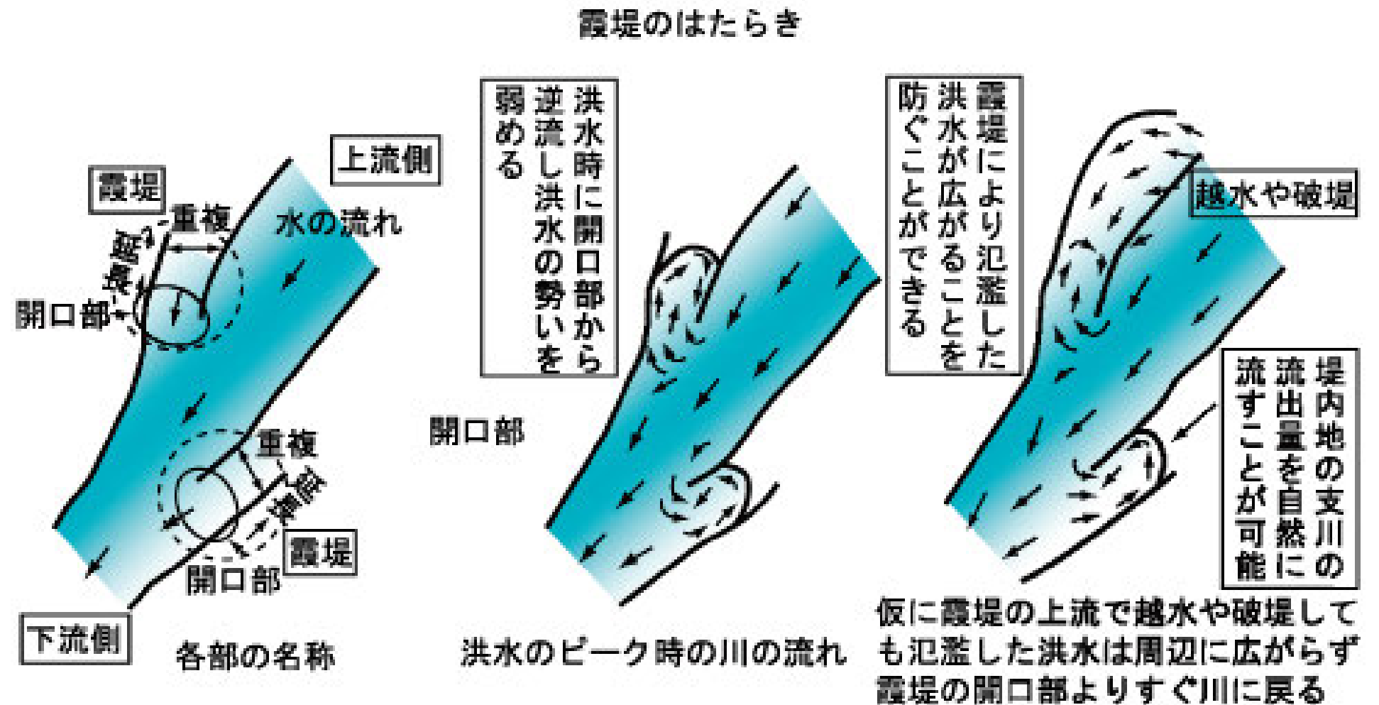
霞堤
