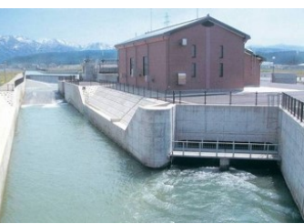
農業用水路を活用した小水力発電施設
