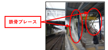
鉄骨ブレースによる耐震補強
