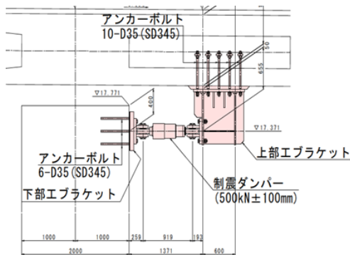
【対策概要: 制震ダンパー概要図】
