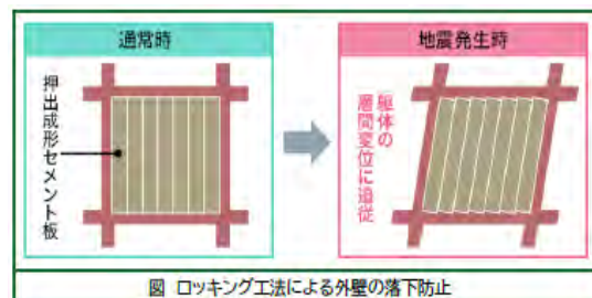
図 ロッキング工法による外壁の落下防止
