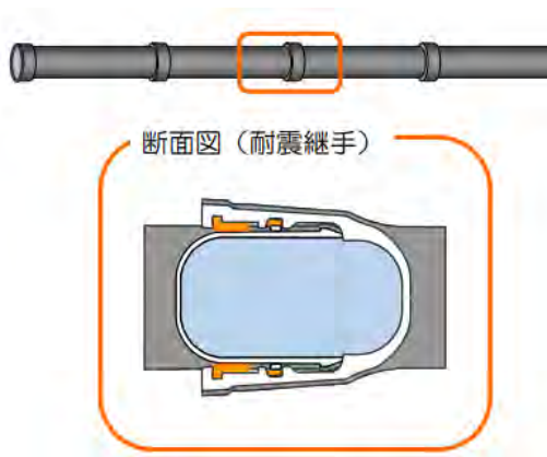
平常時の耐震管
