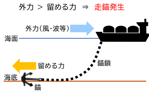
【走錨が発生するメカニズム】
