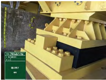
高潮・高波対策(防波堤の倒壊対策等)
