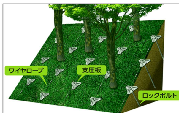
▲ ノンフレーム工法の模式図
