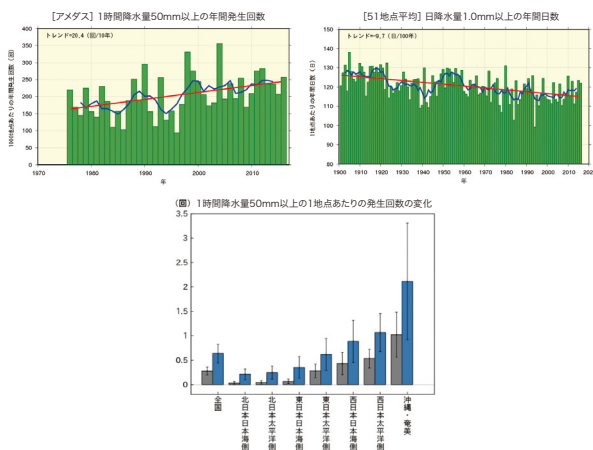
図7 1時間降水量50mm以上の年間発生回数の経年変化(左上)、 日降水量1.0mm以上の年間日数の経年変化(右上)、 1時間降水量50mm以上の年間発生回数の将来変化(下)
