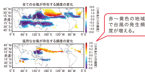
図4 台風の出現頻度の将来予測の一例
