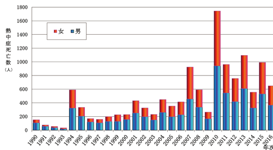
図23 年次別男女別熱中症死亡数（1990～2016年） 出典20より
