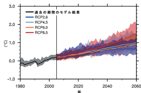
図2 世界の年平均海面水温の将来変化
