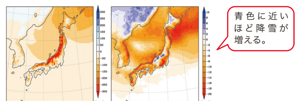
図8 冬季(11月～3月)の総降雪量の将来変化(左)、 10年に一度の大雪(日降雪量)の将来変化(右)の一例
