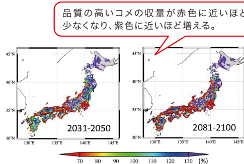
図9 品質の高いコメの収量の変化率分布（適応策をとらない場合の20年平均値で、1981～2000年平均の値を100とした相対値） 出典8より
