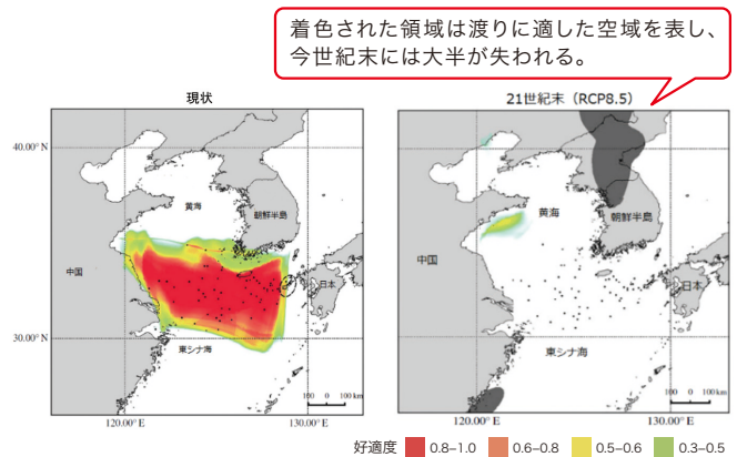
図15 ハチクマの秋の渡りの経路の現状と将来 出典14より一部改変
