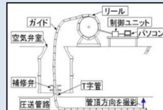
圧送管路腐食調査機器 模式図
