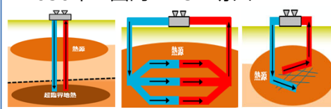
超臨界地熱 クローズドループ EGS
