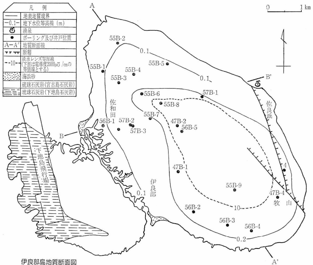
伊良部島地質断面図
