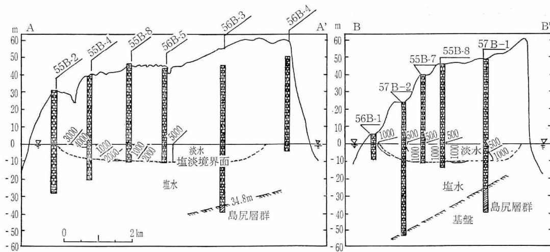
伊良部島・下地島の水文地質図
