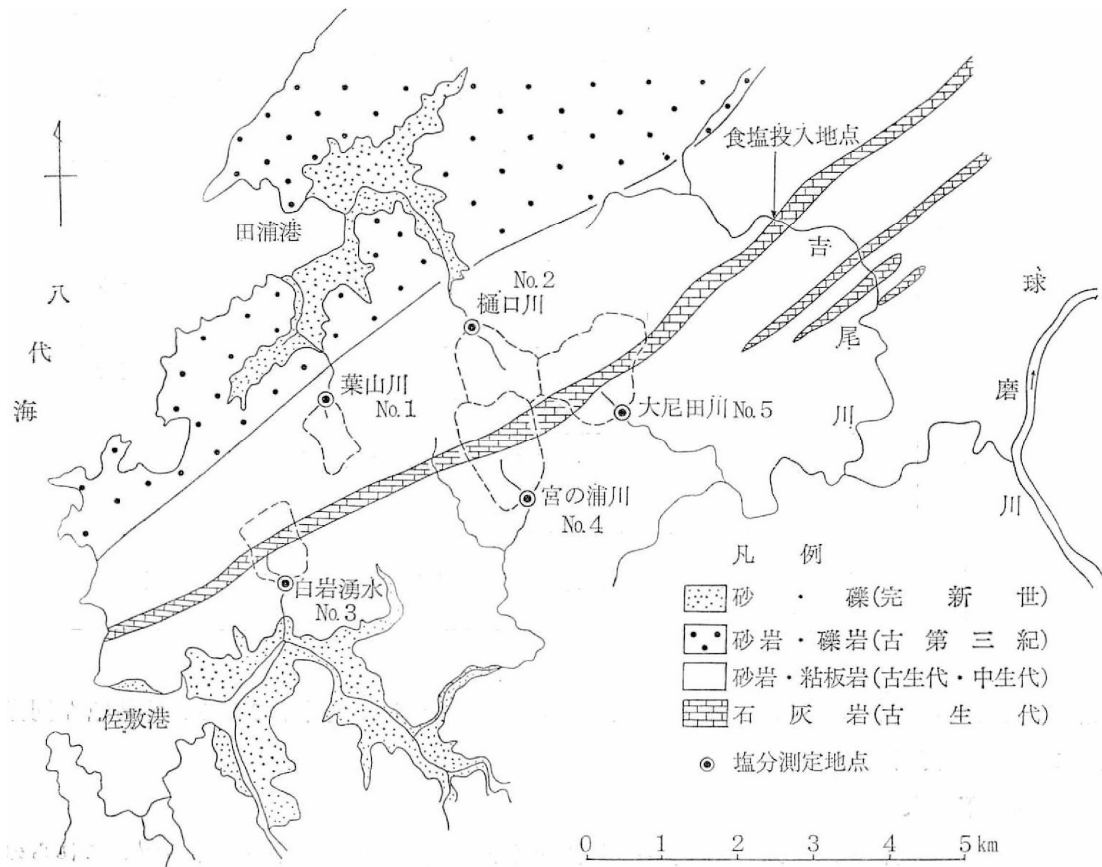
芦北山地地下水流動調査位置図
