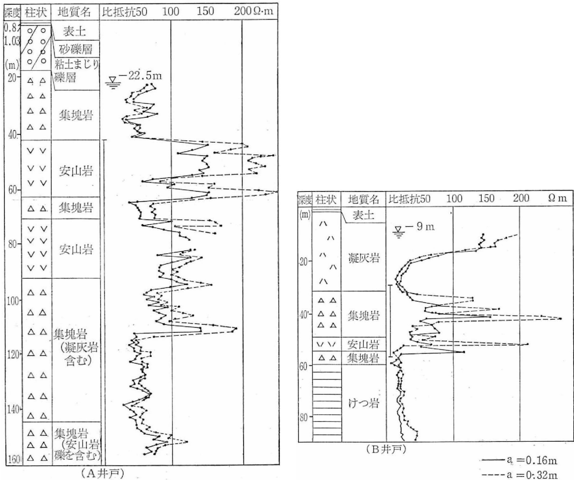
代表的な井戸の柱状図
