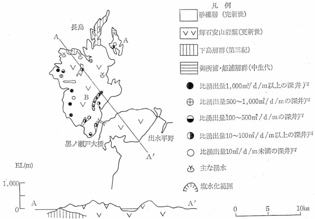
長島の水文地質図
