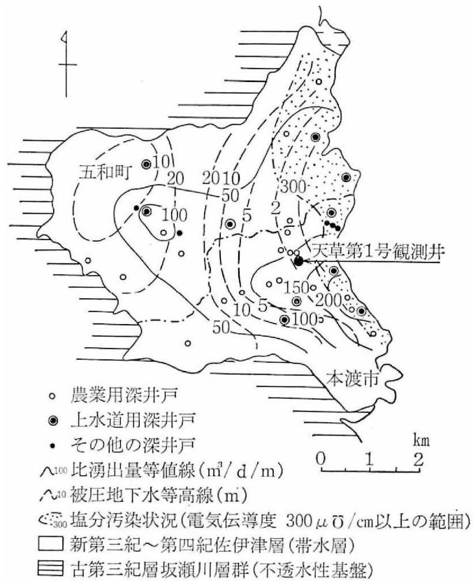
天草下島佐伊津地域の水文地質図
