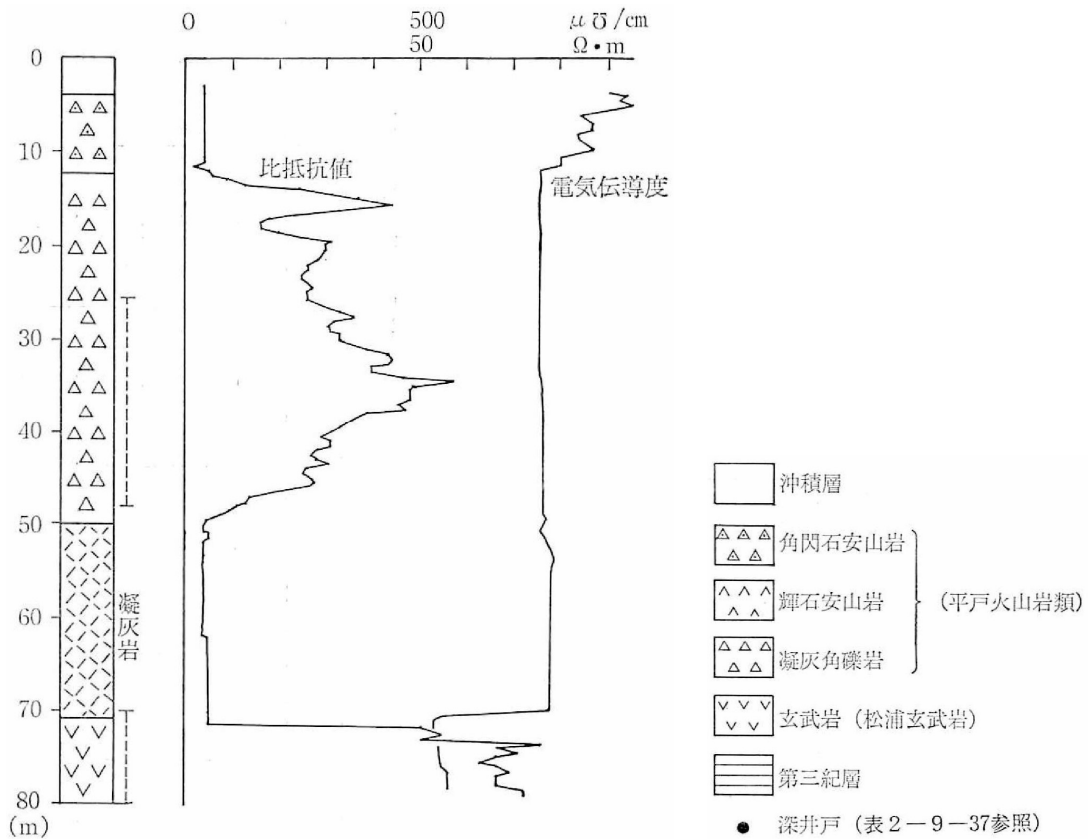
No.1 号井地質柱状図
