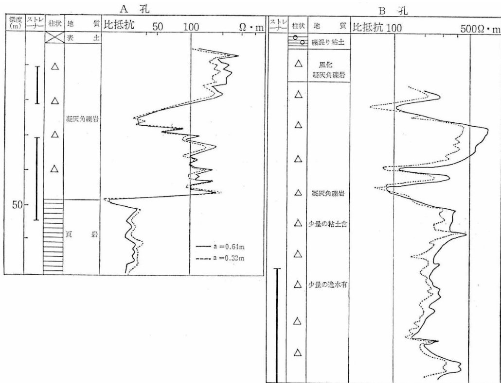
代表的なさく井柱状図
