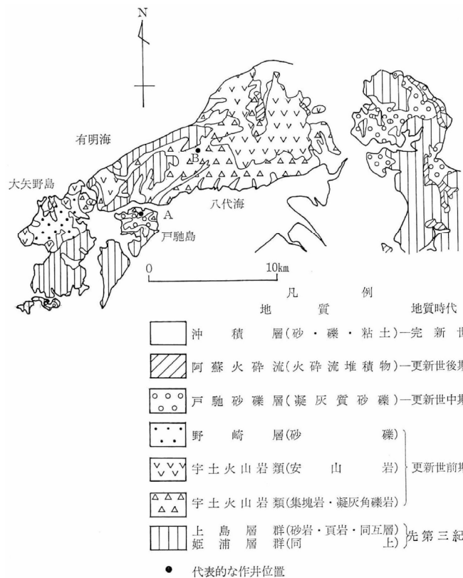
三角半島の地質図
