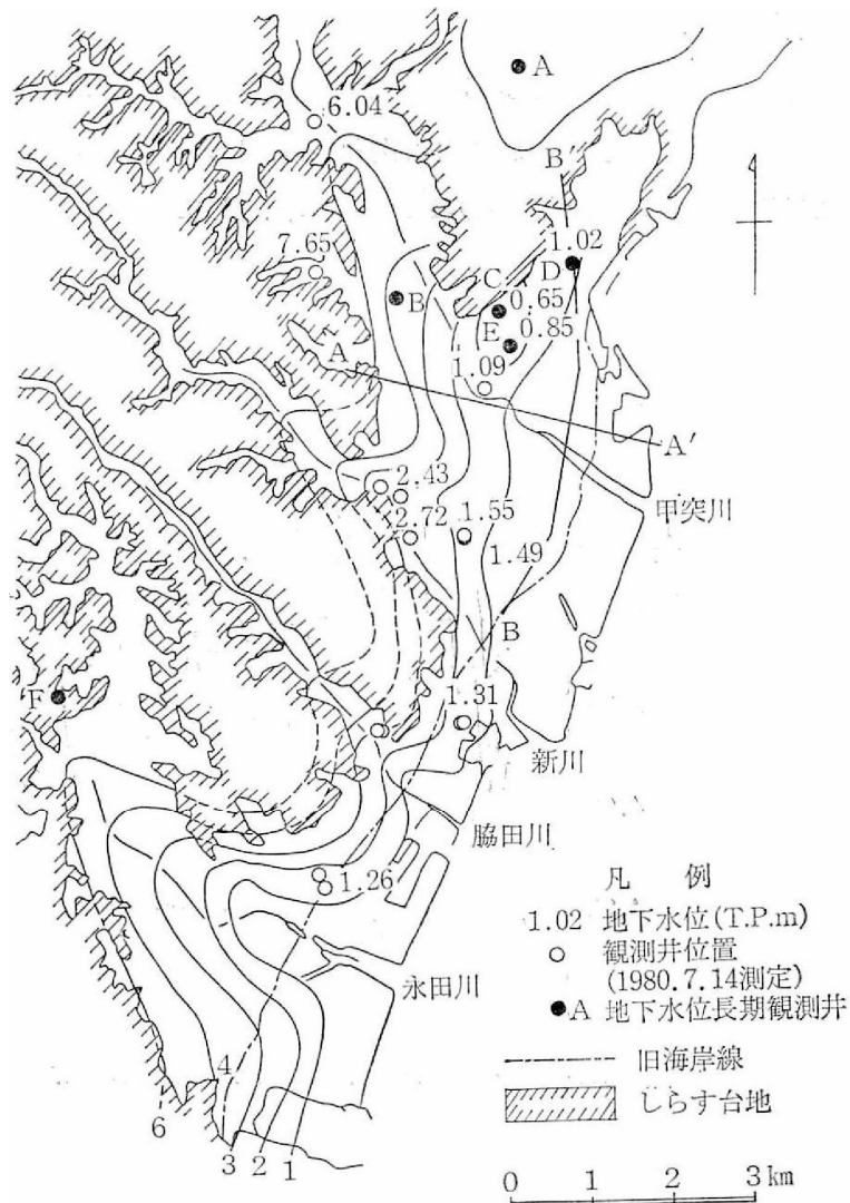
地下水面図
