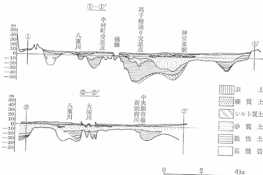
地質断面図
