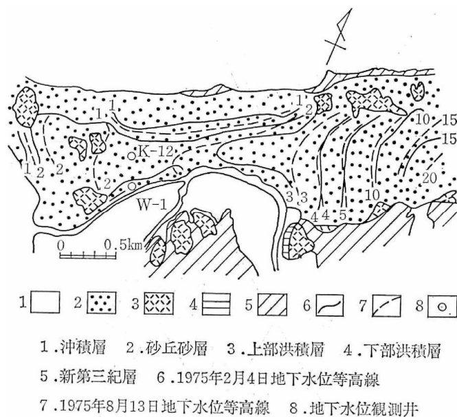
久美浜砂丘の水文地質概要図
