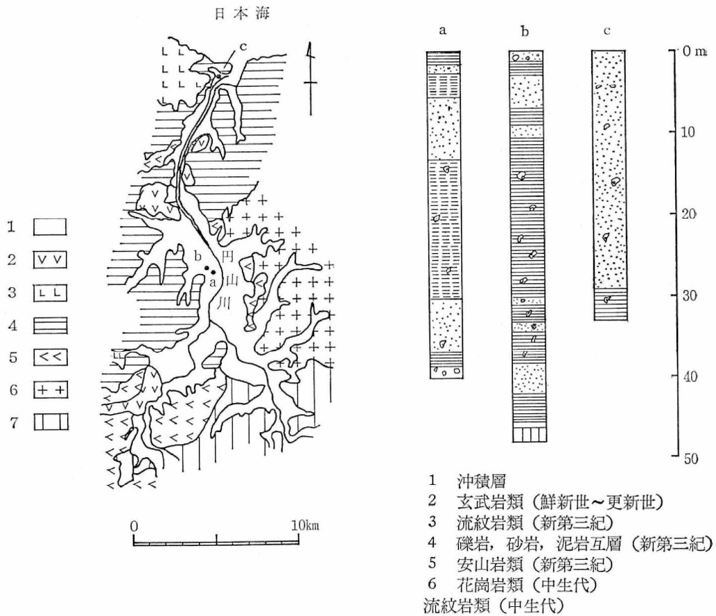
豊岡盆地の地質図および地質柱状図
