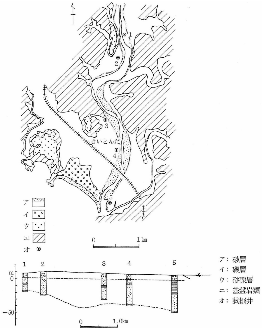
富田川沿岸の地質概要図
