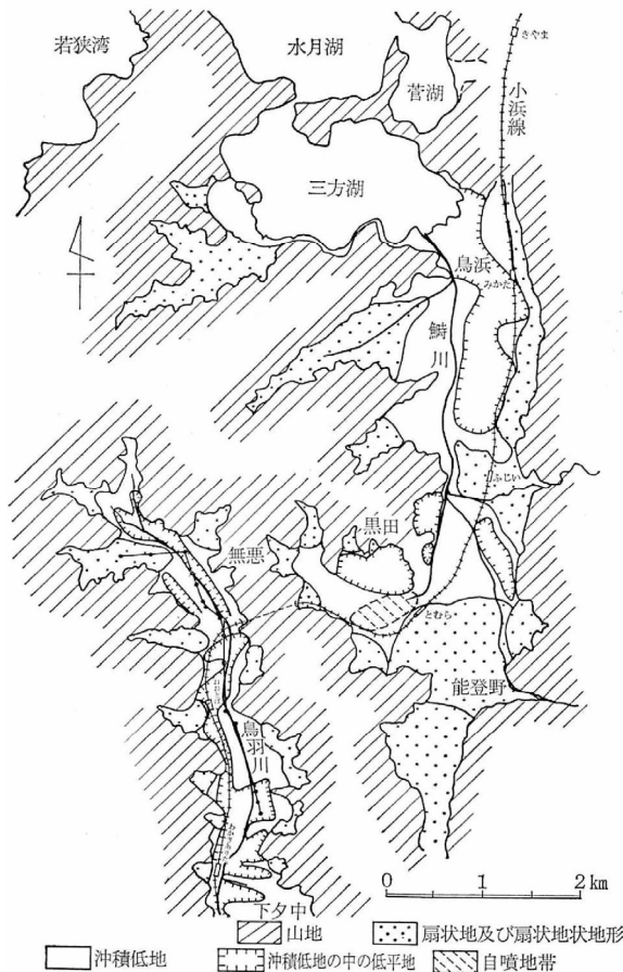
鱒川・北川支流鳥羽川沿いの微地形区分図
