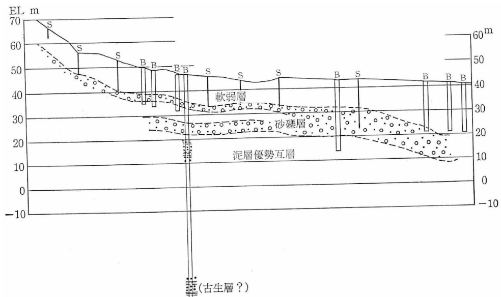
鳥羽川流域の模式断面図
