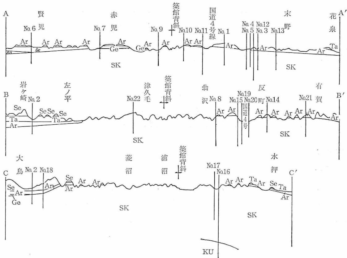
水文地質断面図
