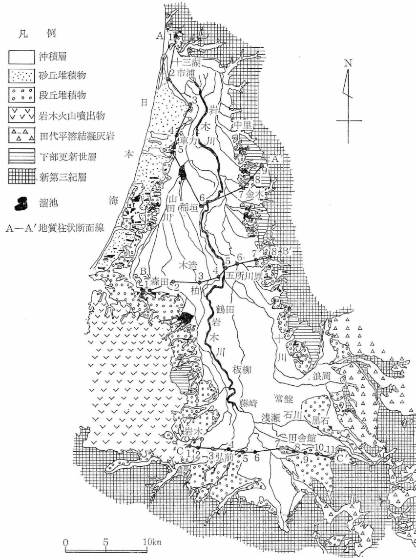
津軽平野の地質図
