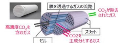
【新規分離膜の開発例】
