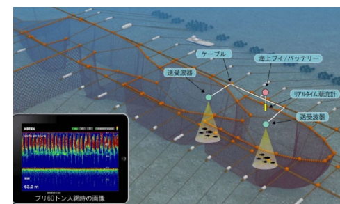
遠隔式魚群探知機 （日東製網（株）より提供）
