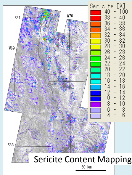
資源探査に資する鉱物の分布図
