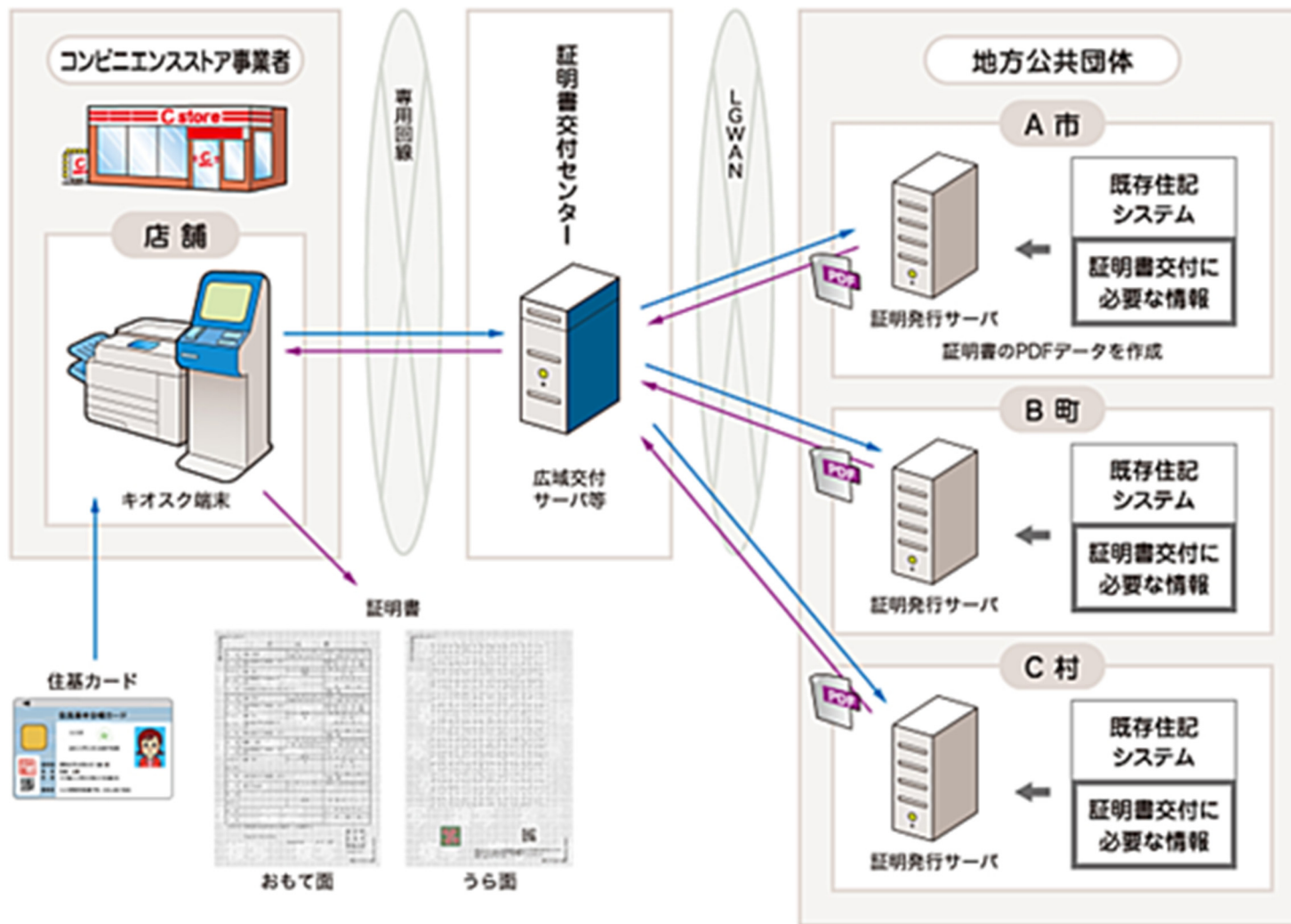
図3 コンビニエンスストアにおける証明書交付のシステム構成イメージ 出所: 地方自治情報センターホームページ ( http://www.lasdec.nippon-net.ne.jp/cms/9,15011,93.html ) より
