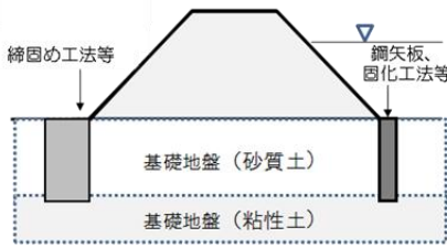
堤防の液状化対策(例)
