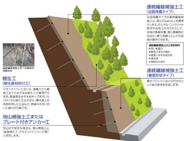
▲ジオファイバー工法の模式図
