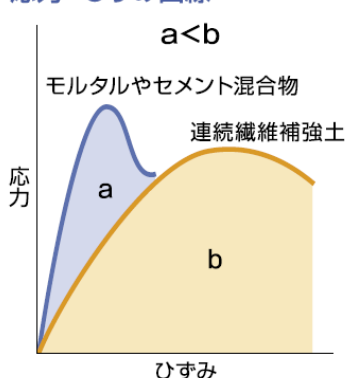
応力-ひずみ曲線
