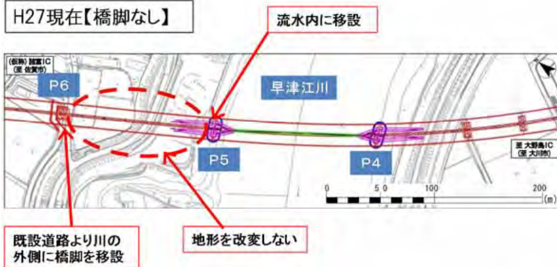
図7 橋脚位置の見直し
